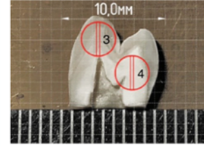
Рисунок 2. Образец №2, точки приложения антенны эхо-импульсного пьезопреобразователя 3, 4.
